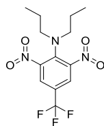
Trifluralin
