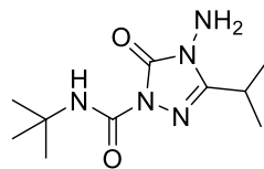
Amicarbazone
