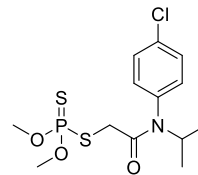
Anilofos
