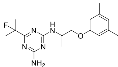
Triaziflam
