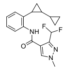
Sedaxane 2011
