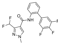
Fluxapyroxad 2011
