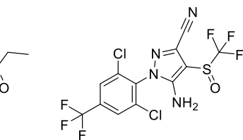
Ethiprole
