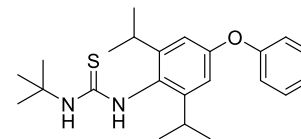
Diafenthiuron
