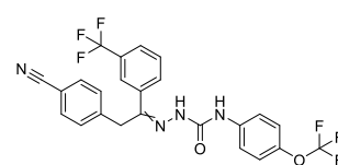
Metaflumizone
