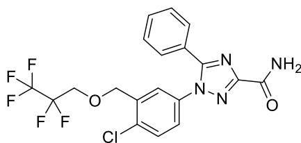
Flupoxam
