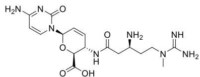
blasticidin S
