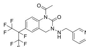
Pyrifluquinazon
