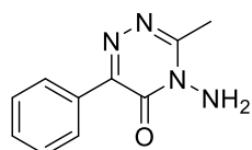
Metamitron
