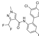
Bixafen 2011
