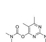
Metolcarb
