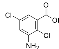
Chloramben
