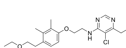
Pyrimidifen
