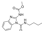
benomyl
