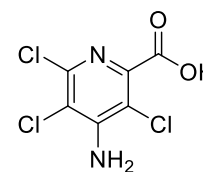
Picloram
