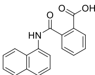
Naptalam
