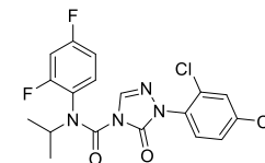
Ipfencazone
