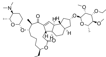
Spinetoram
