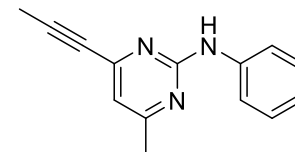
mepanipyrim
