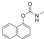
Carbaryl
