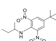
Norflurazon
