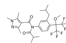
Pyflubumide
