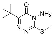
Metribuzin
