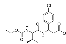
valifenalate
