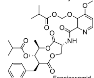
Fenpicoxamid
