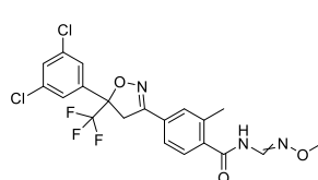
Metaflumizone
