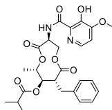
(+)-UK-2A
