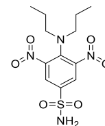
Oryzalin
