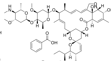
Emamectin
