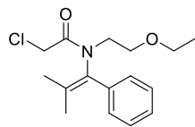
Pethoxamid
