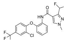
Flubeneteram 2020
