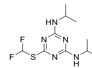
Fucaojing
