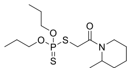
Piperophos
