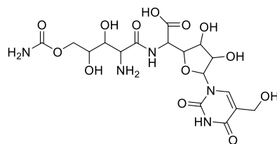
polyoxin
