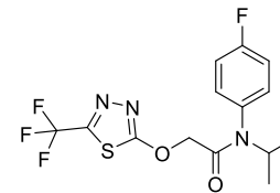
Flufenacet
