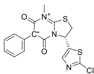
2413390-32-4 双噻唑(fenmezoditiaz)
