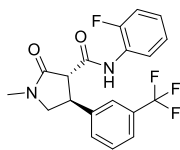
2053901-33-8 tetflupyrolimet
