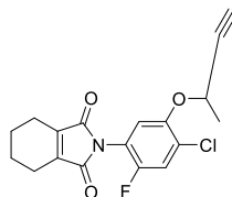
炔草胺(flumipropyn)
