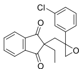
茚草酮(indanofan)
